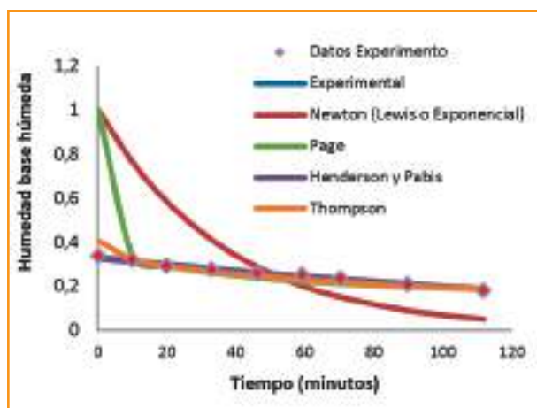
Figura 9: Comparación de curvas de secado experimental con algunos modelos matemáticos en el secador de bandejas a 40°C (Muestra 2)
